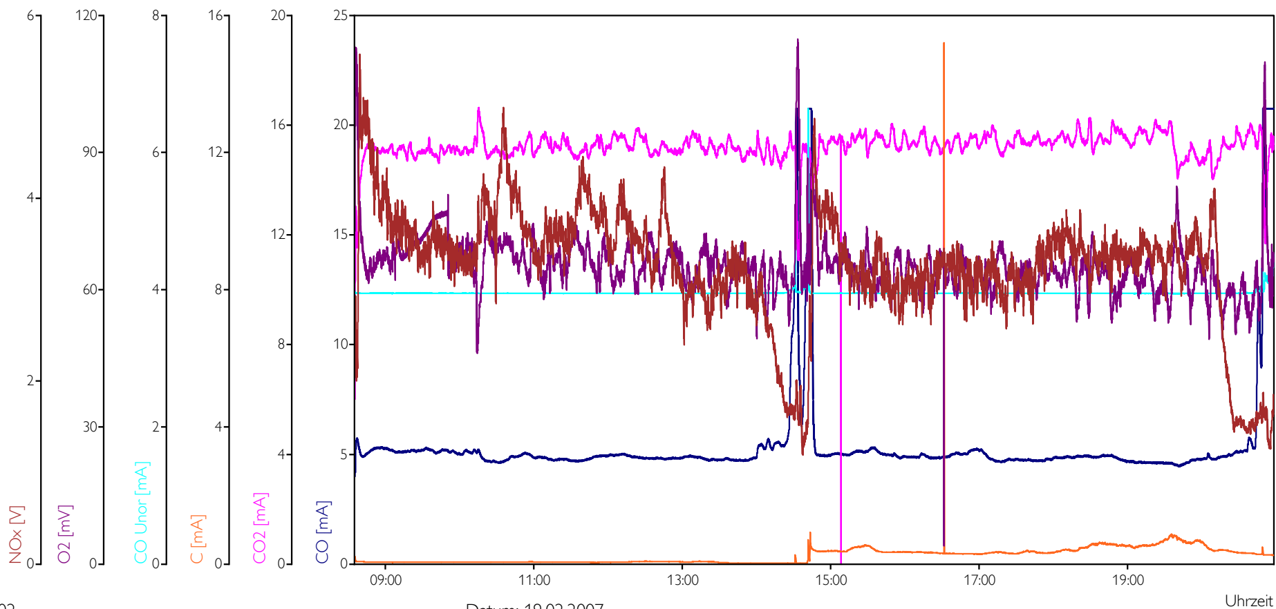
Typenprüfung ÖNORM EN 303-5 - Rohdaten Konzentrationsverlauf
